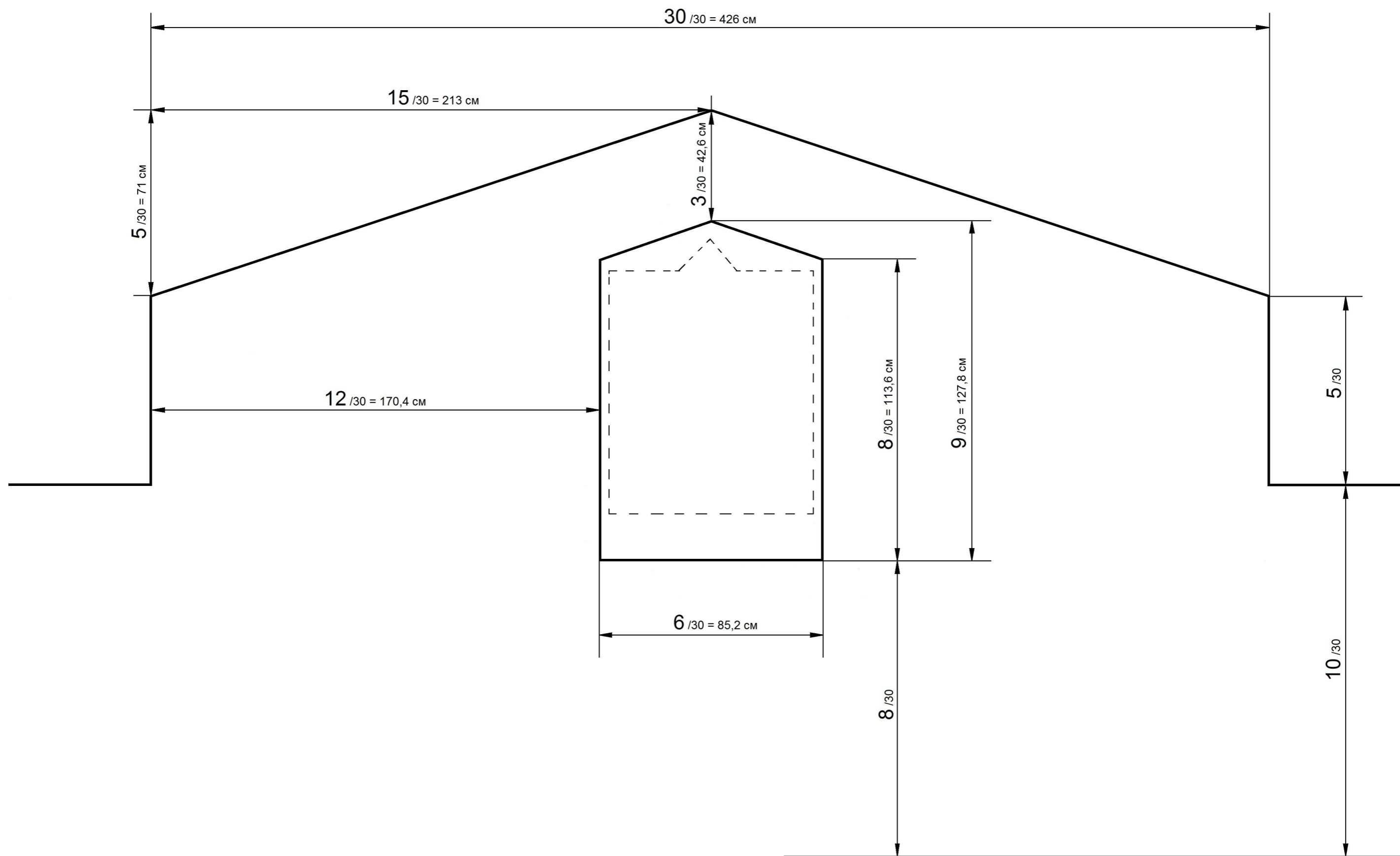
Схема размещения бронзовой доски на мемориальной стене памятника Затопленным кораблям.
